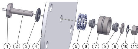
Pokrywa kołnierzowa 6 mm
