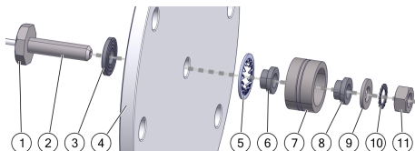
Pokrywa kołnierzowa 8 mm
