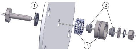
* Abbildung Zahnscheiben, Montagetopf ggf. abweichend
