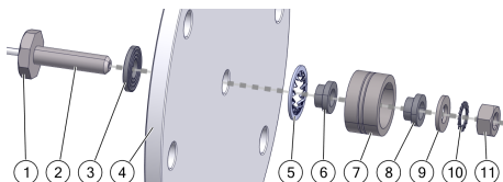
Flanschdeckel 8 mm
